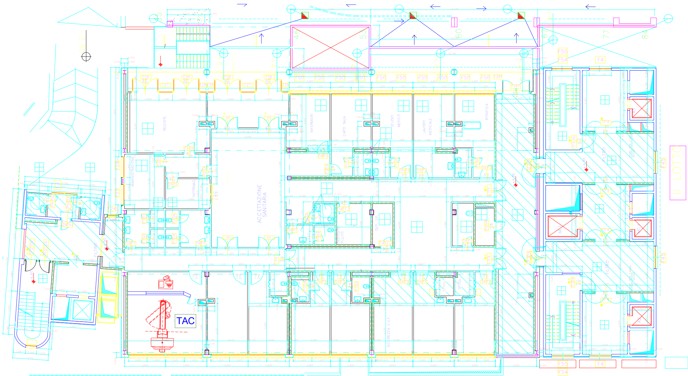
QUARTO LIVELLO NUOVO EDIFICIO D.E.A. PRESIDIO OSPEDALIERO "ANNUNZIATA" DI COSENZA
